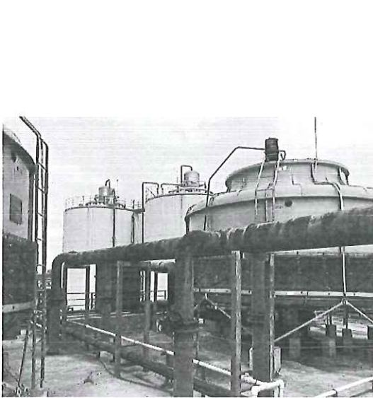
渗滤液处理站设备设施锈蚀情况
